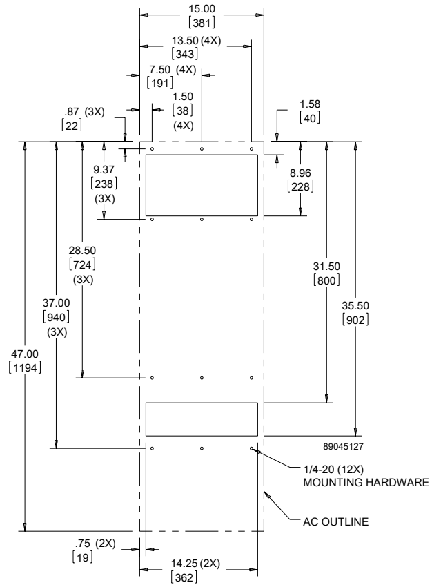
Cutout Dimensions
